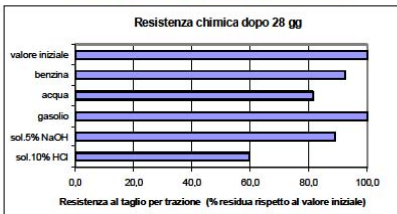
Resistenza al taglio per trazione dopo immersione in vari mezzi (ASTM D1002)
